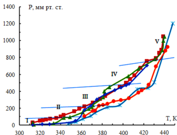
Рисунок 2 - Барограмма процесса термического разложения \text{Th}(\text{NO}_3)_4 \cdot 5\text{H}_2\text{O} Figure 2 – Barogram of the thermal decomposition process
