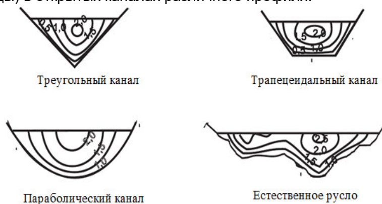
Рисунок 2 – Типичные распределения скоростей течения жидкости (воды) в открытом канале Figure 2 – Typical flow velocity distributions of fluid (water) in an open channel
