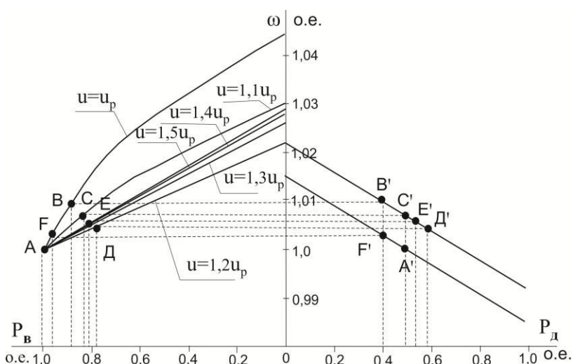
Рисунок 1 – Распределение активной мощности между ветроагрегатом с регулированием угла разворота лопастей и дизелем при P_0:P_n=1:1 и u \geq u_p
